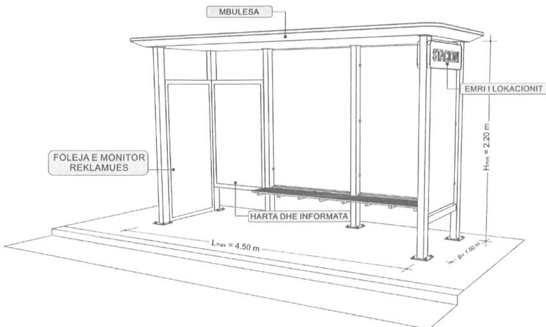
Figura 2: Kabina për pritje të autobusit, sipas pozicionit nr. 6 të paramases
