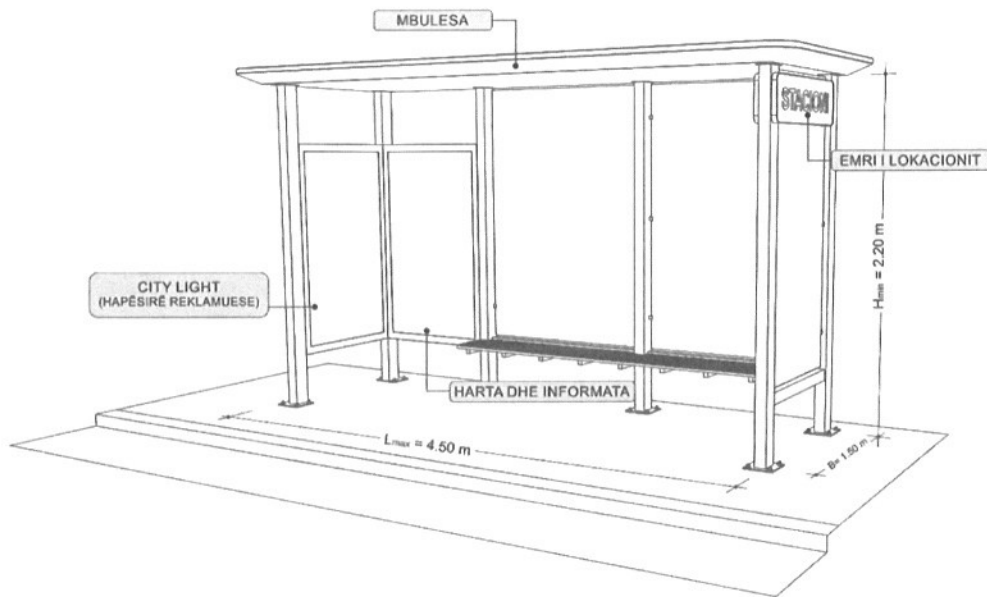
Figura 1: Kabina për pritje të autobusit, sipas pozicionit nr. 5 të paramases
