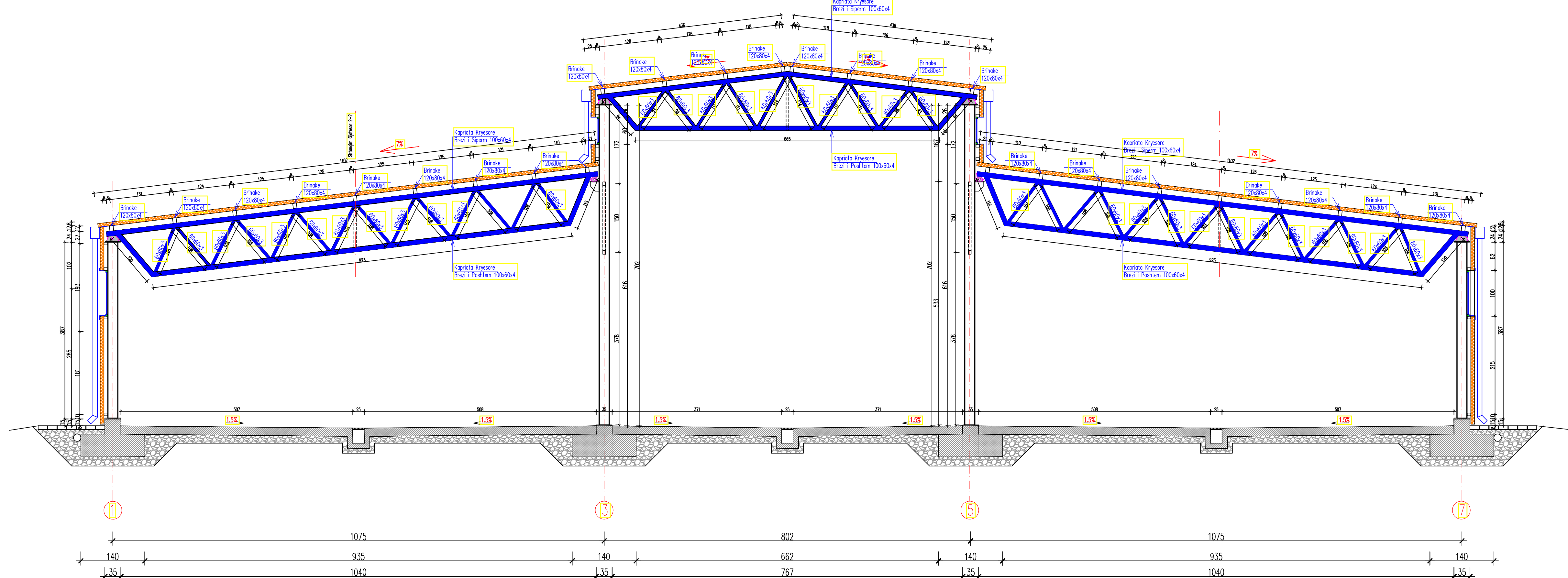
Prerja Terthore c-c
