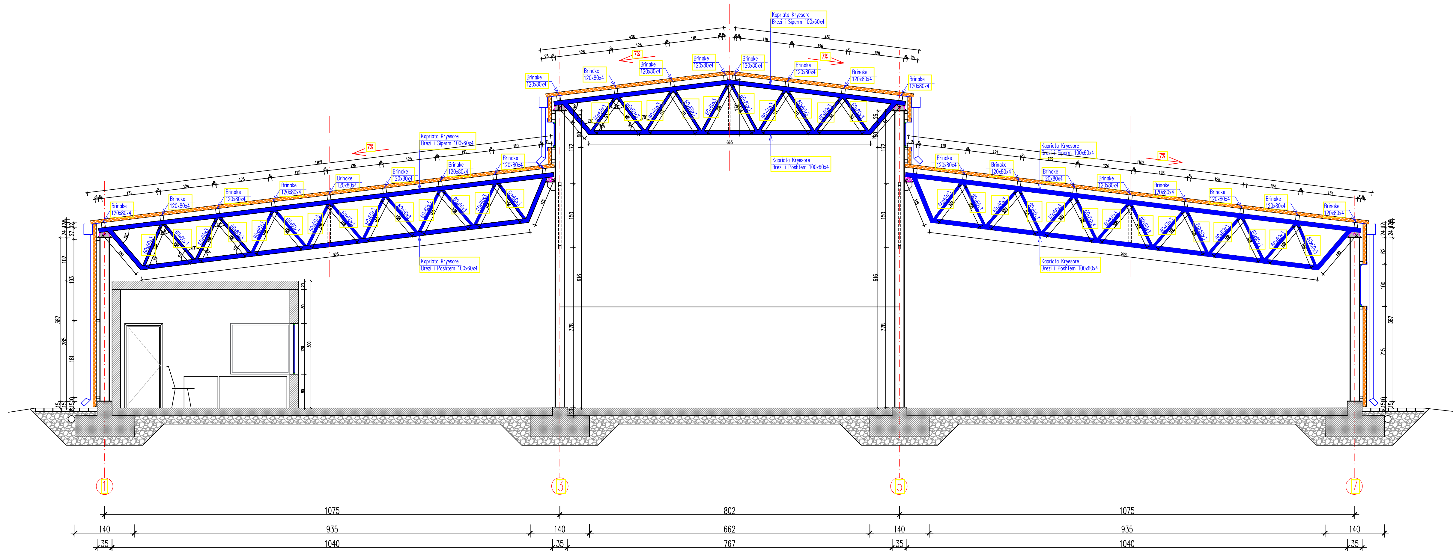
Prerja Terthore b-b
