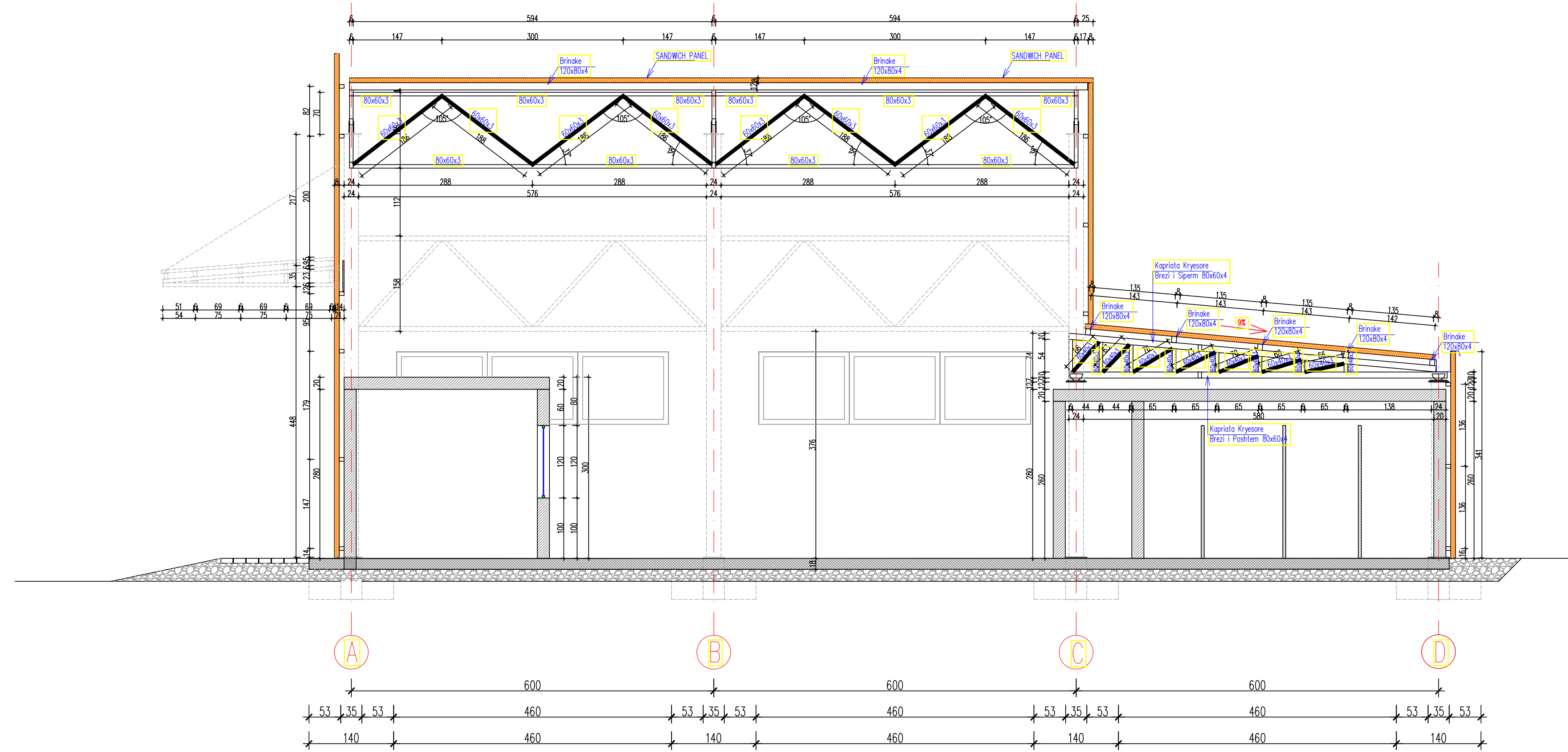
Prerja Gjatesore d-d
