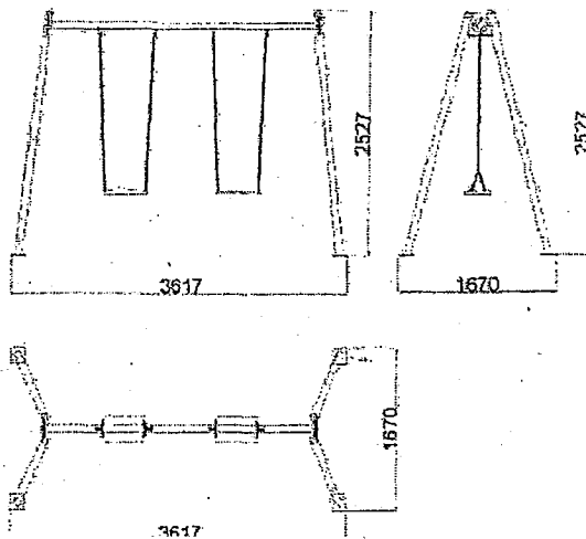
Rekuizita : Steel Swings -135 kg , Fig.14/1
