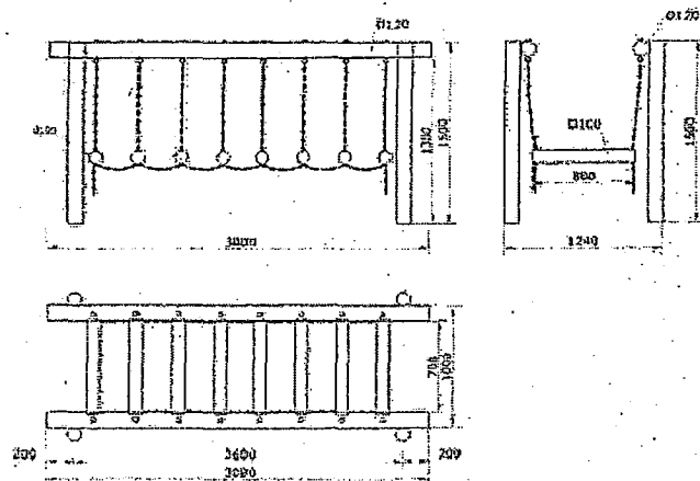
Rekuizita : " Balancing 108 kg ", Fig.20 / 1
