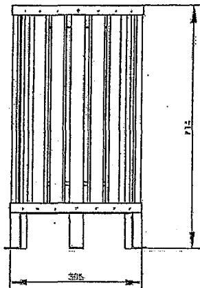
Shtëpi për mbeturina : Fig. 5 /1
